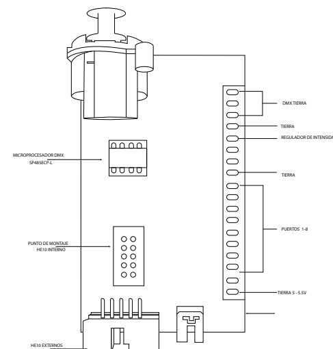
DIAGRAM DE TARJETA INTERNA
