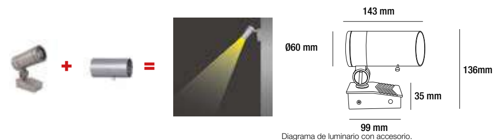
Diagrama de luminario con accesorio. *Accesorio se vende por separado
