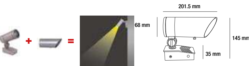
Diagrama de luminario con accesorio. *Accesorio se vende por separado
