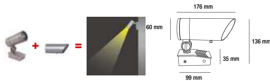
Diagrama de luminario con accesorio. *Accesorio se vende por separado
